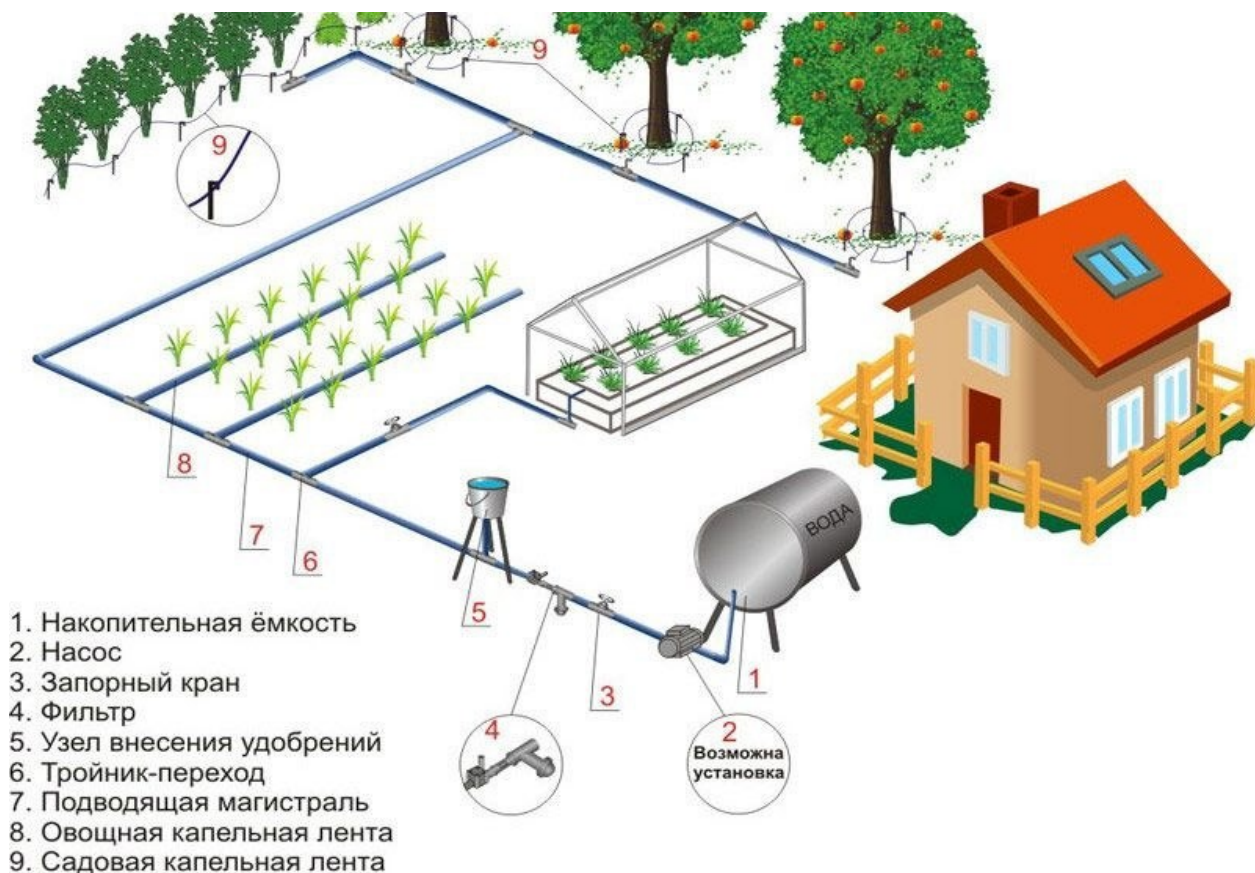
Рисунок 2 - Общая схема системы капельного полива
